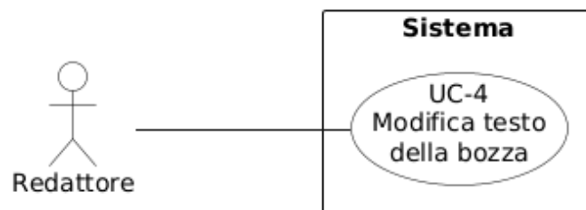
Figura 11: Diagramma del caso d'uso UC-4: Modifica testo della bozza
