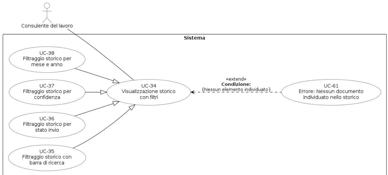
Figura 48: Diagramma del caso d'uso UC-34: Visualizzazione storico con filtri
